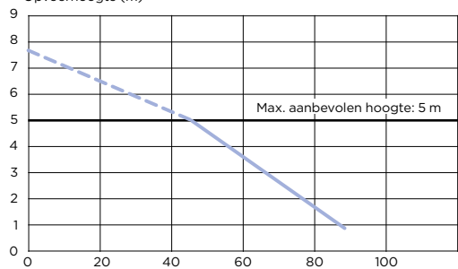
Opvoerhoogte (m)
