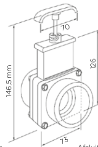
Afsluiter met diameter 50
