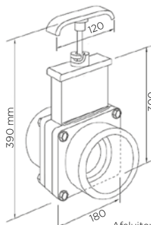
Afsluiter met diameter 110 of 100 mm
