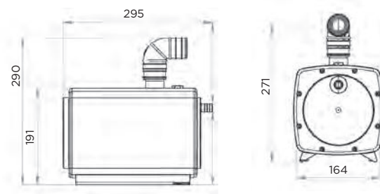
Dimensions de la pompe
