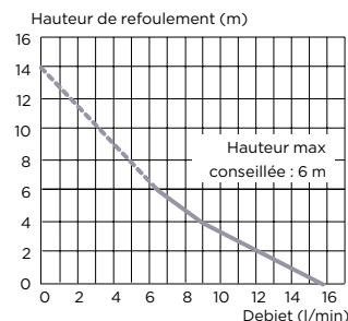
Sanicondens Clim mini (livré avec une plaque de fixation)
